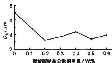
图 1 超细重钙粒子粒径与聚羧酸钠盐分散剂加入量之间的关系
