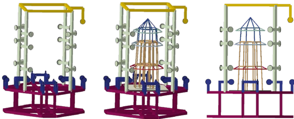
(a) 加载架示意图 (b) 模型安装效果图 (c) 模型安装后侧视图
